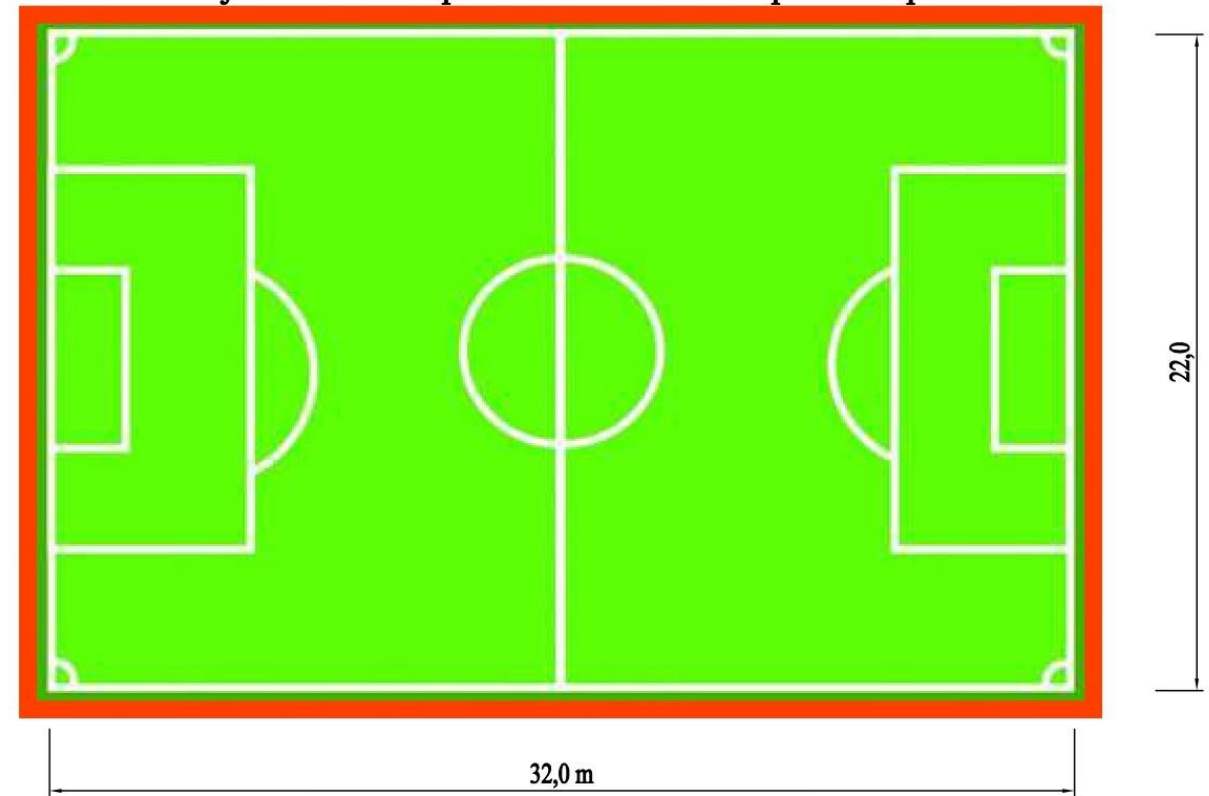
Amenajarea terenului sportiv de mini-fotbal în parcul de pe str. Mateevici
